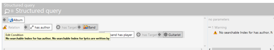
Strukturabfrage mit Rückmeldung zu fehlender Indexierung
